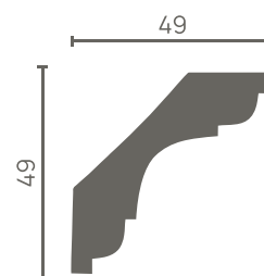
DD05 — 49x49x2000 mm
