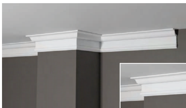
DD501 — 59x31x2000 mm
