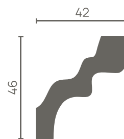
DD39 — 46x42x2000 mm
